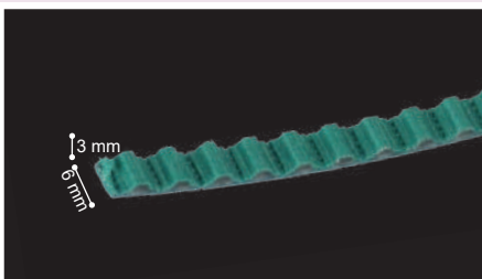
Correa dentada RS10
