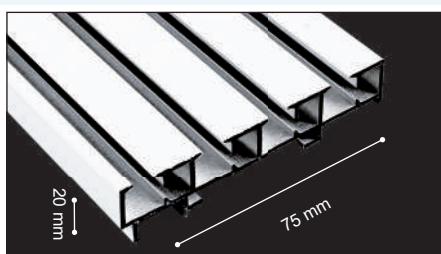
Perfil de Aluminio 4 vías (75x20mm)
