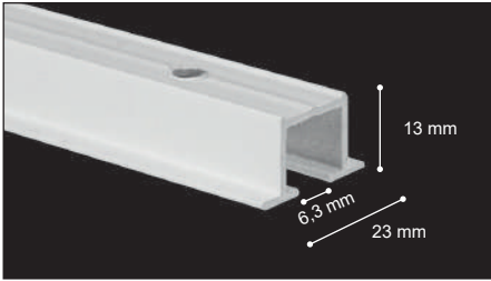
Perfil con agujeros /Track with holes /Rail avec trous
