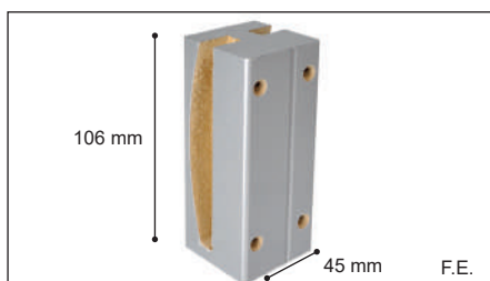
Empalme Splice / Raccordeur
