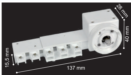
Tapa MOTOR Panel Japonés Motorizado 5 vías
