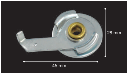
Soporte Techo Giratorio
