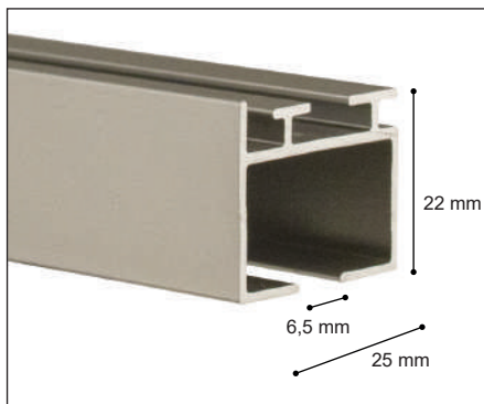
Perfil Cascais® Inox /
