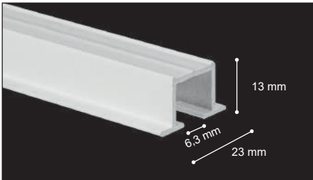
Perfil sin agujeros /Track without holes /Rail sans trous
