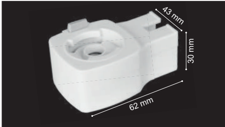
Cantoneira motriz RS10
