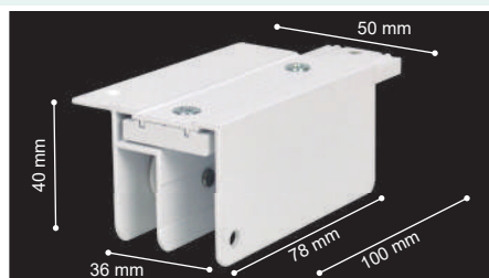
Juego Cantonera para cordón
