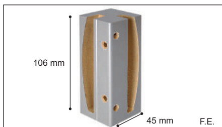
Codo esquina Outer joint / Coude extérieur
