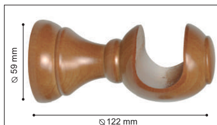
Soporte Madera Clásico 30 mm
