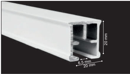
Riel RS10 motorizado
