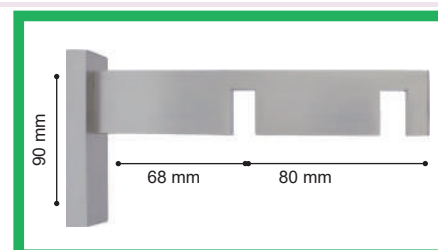
Soporte Doble Pared
