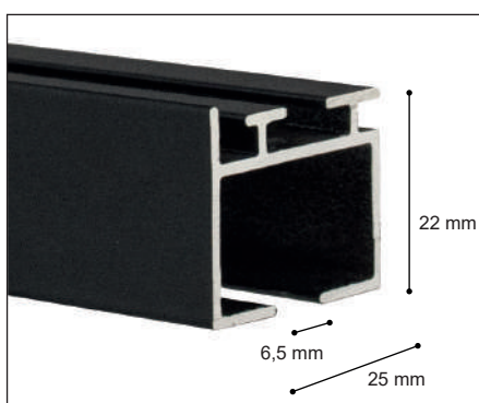
Perfil Cascais® Negro /
