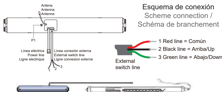
Esquema de conexión Batería Externa
