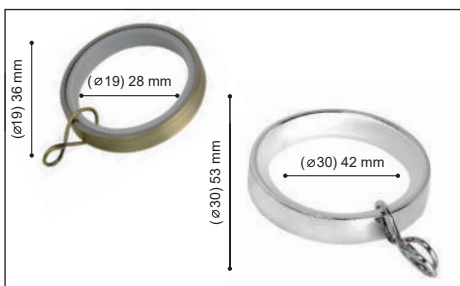
Anilla Plana con teflón
