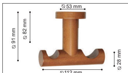
Soporte Madera Techo Doble
