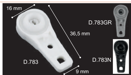
Corredera con Ruedas
