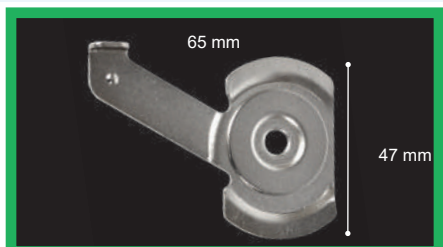
Soporte Panel Japonés Motorizado
