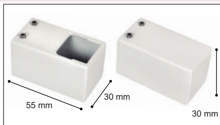
Terminal Tapón Sintra® (Sistema Cordon)
