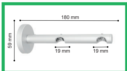
Soporte Doble Pared 19/19mm
