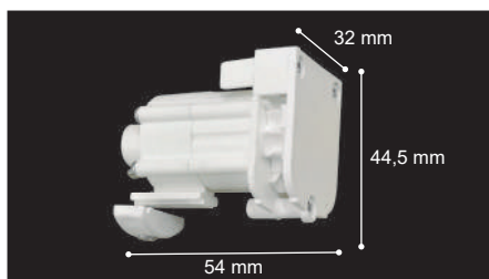
Freno 1:4 (sin cadena)
