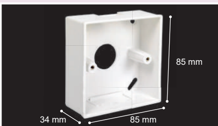
Caja para empotrar Receptor Pulsador /
