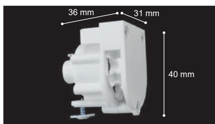
Freno 1:1 (sin cadena)
