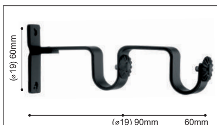
Soporte Pared Doble
