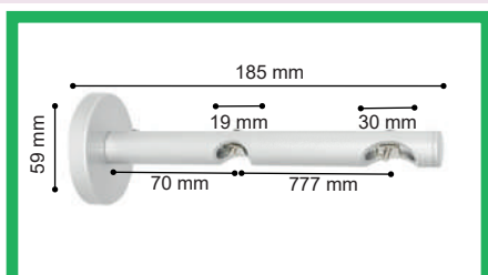
Soporte Pared 30/19 mm
