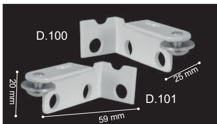
Soportes laterales Soportes laterales
