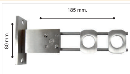
Soporte Técnico Doble 19/19
