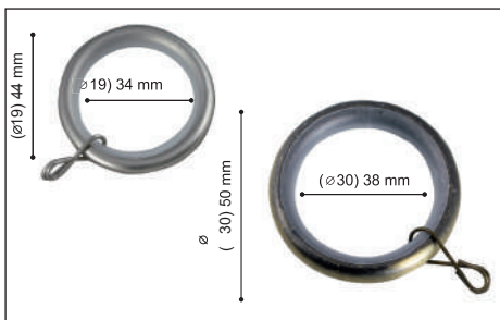
Anillas con Teflón
