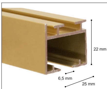
Perfil Cascais® Dorado /
