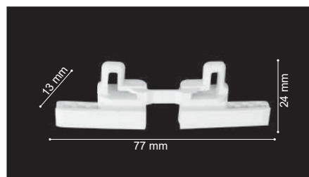
Bloca correa RS10
