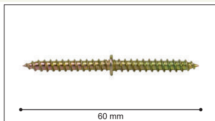
Dowell de Empalme 60 mm x 5 mm
