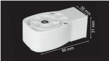
Cantoneira retorno RS10
