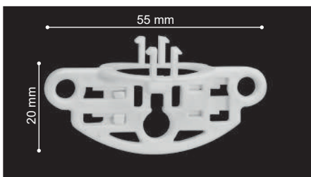
Cierre y freno onda perfecta. Aplicable a: D.113, 114, 117 y 118
