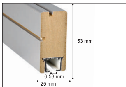
Perfil Capri Capri Profile / Capri Rail
