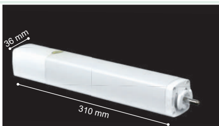
Motor RM09-40B Bateria
