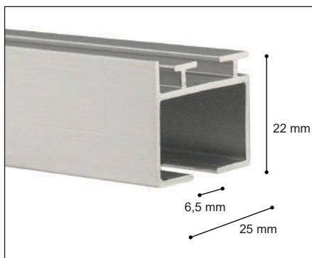
Perfil Cascais® Plata Gratada /
